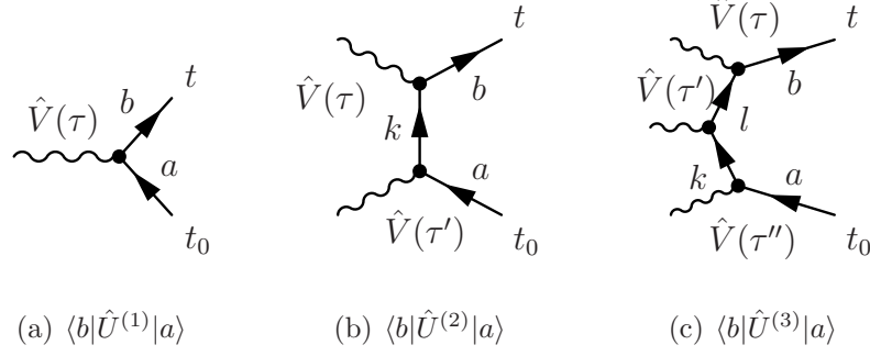
FIG. 12.1. Feynman diagrams
